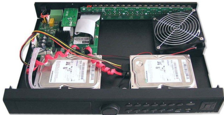
Устройство видеорегистратора – установлено 2 жестких дисков
